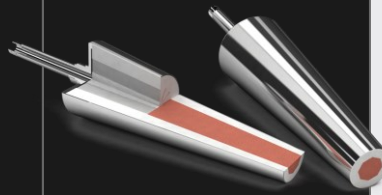
Kształtki gazoprzepuszczalne
